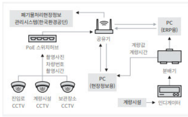
폐기물처리현장정보 시스템 구축도
